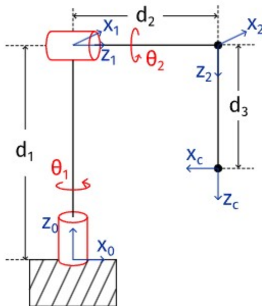
Furuta Pendulum
